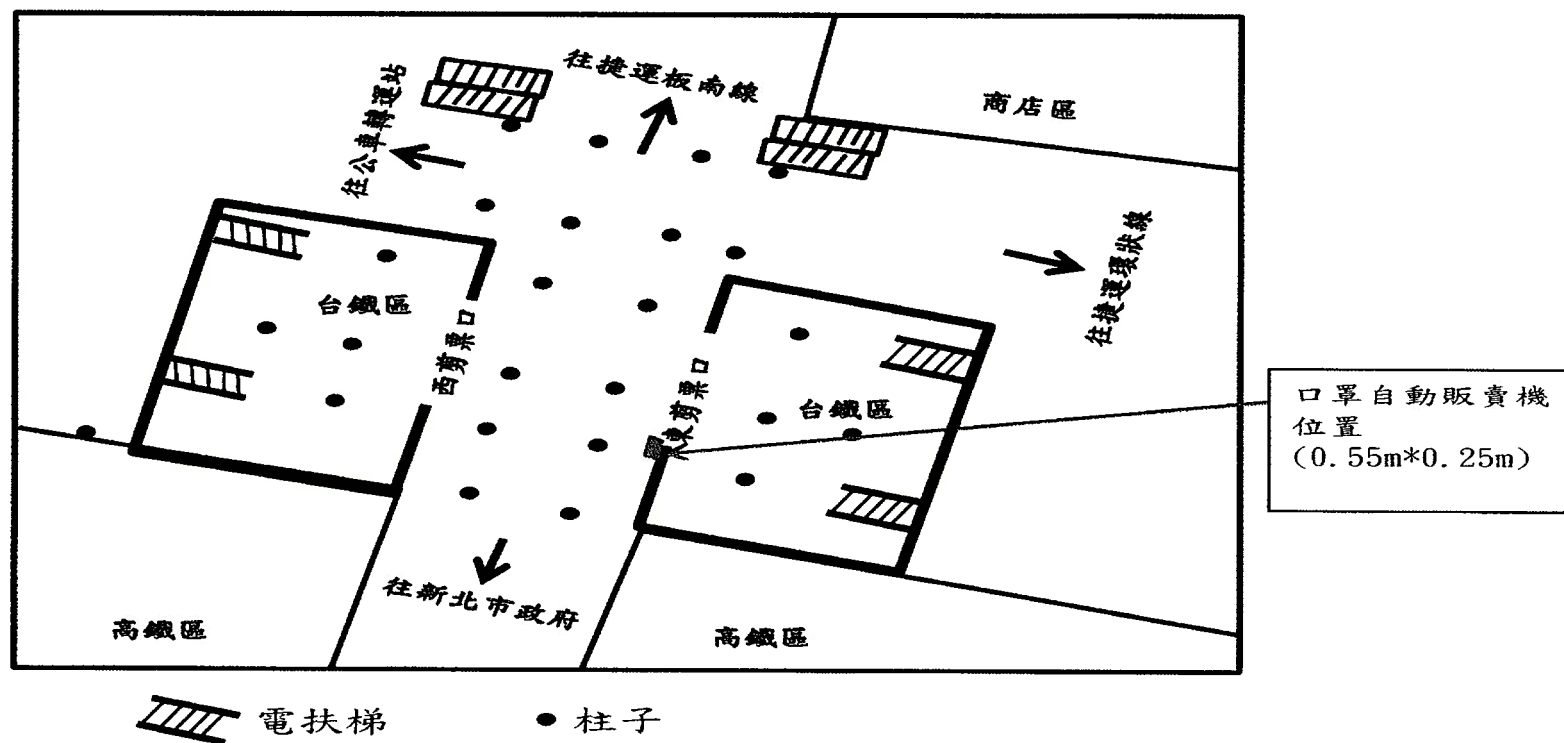
臺鐵板橋車站地下 1 樓平面圖
