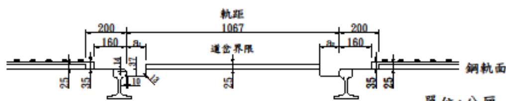
a 1 及a 2 部分之界限詳圖
