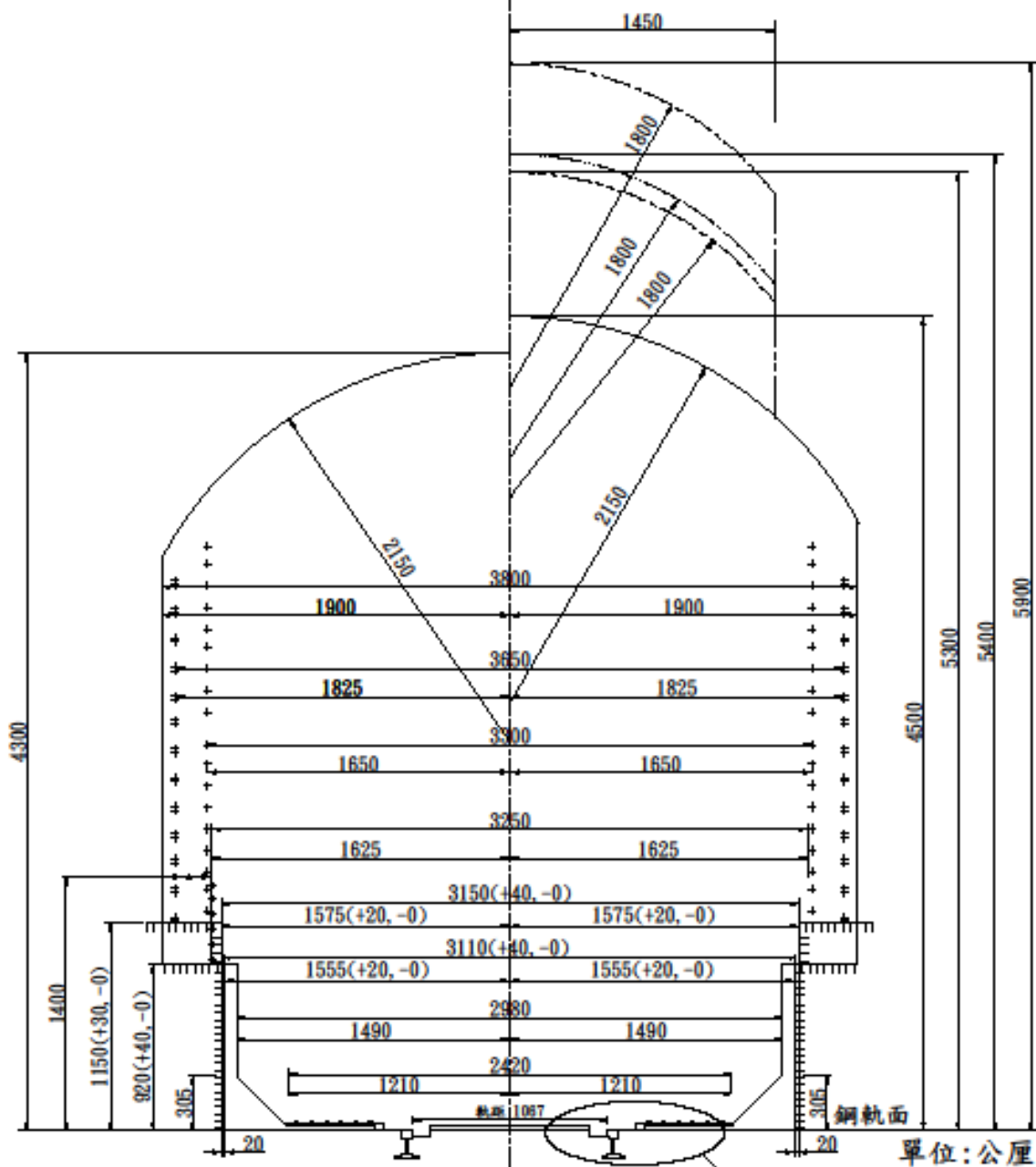
一般路線建築界限圖
