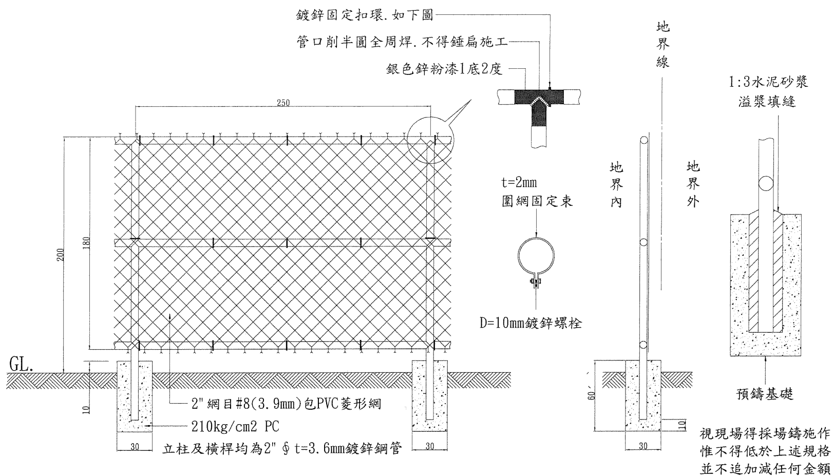
TYPE A 菱形網圍籬施工詳圖 S:1/25
