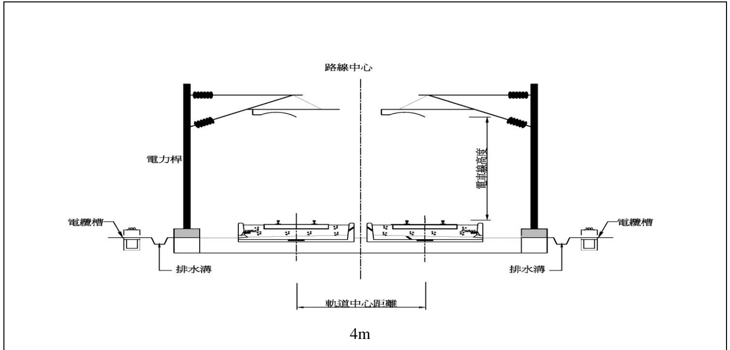
圖 4 軌道斷面圖
